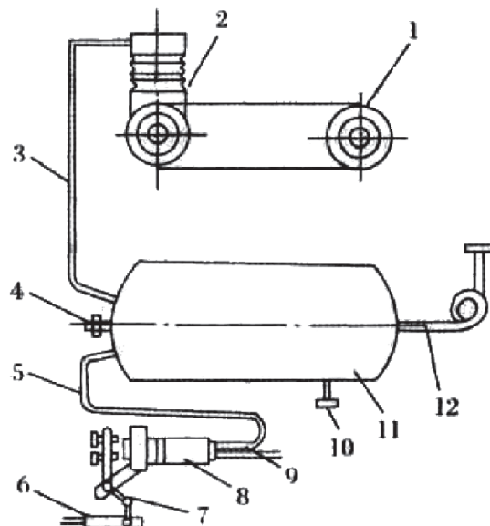
Рис. 3.18. Структура пневмотормоза.
